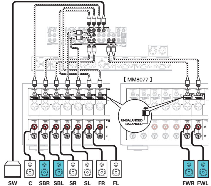
[Anschlussbeispiel] UNBALANCED RCA-Anschluss
