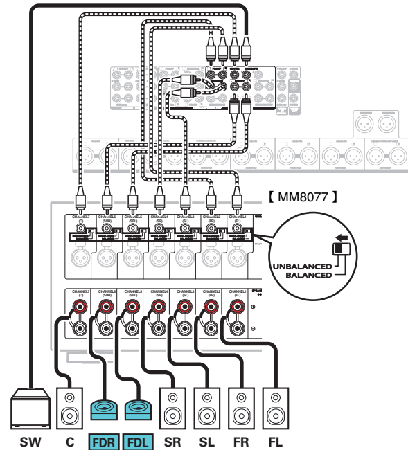
[Anschlussbeispiel] UNBALANCED RCA-Anschluss
