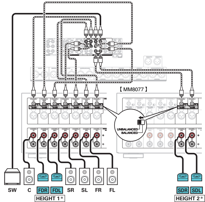
[Anschlussbeispiel] UNBALANCED RCA-Anschluss
