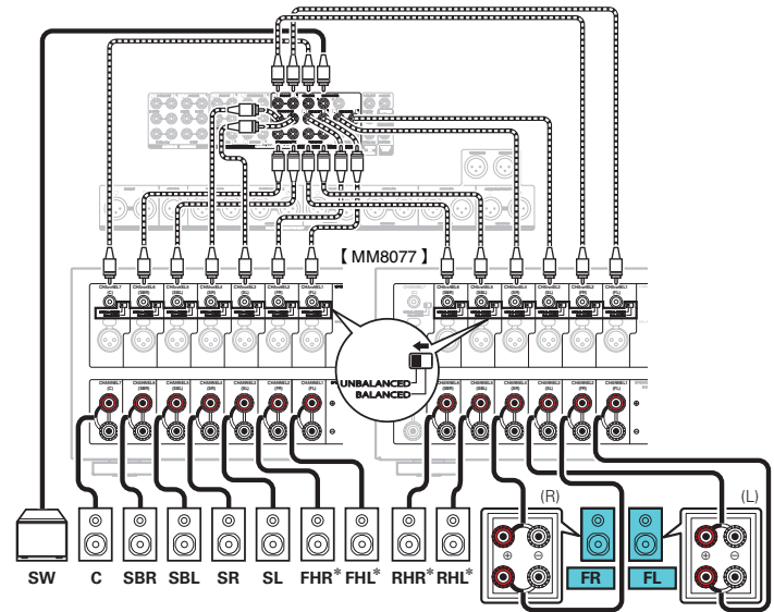
[Anschlussbeispiel] UNBALANCED RCA-Anschluss
